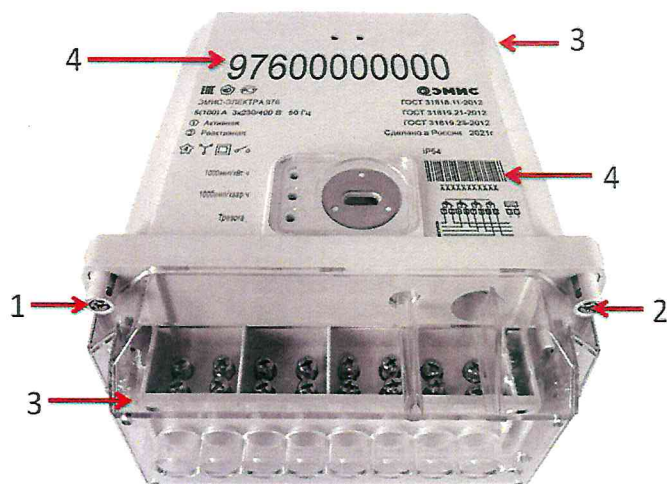
Рисунок 1 – Общий вид счетчика исполнения «С» со схемой пломбировки
